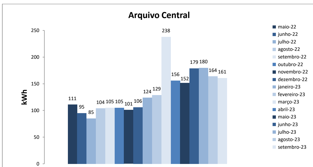
Figura 1. Variação do consumo de energia elétrica da edificação do Arquivo Central.
