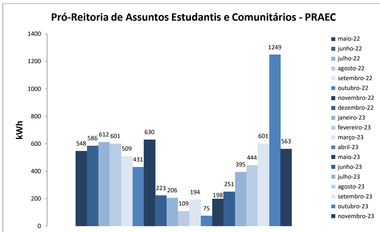
Figura 1. Variação do consumo de energia elétrica da edificação da PRAEC.
