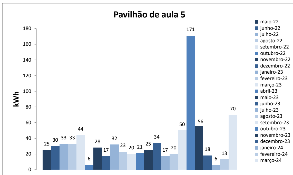
Figura 1. Variação do consumo de energia elétrica da edificação do Pavilhão de Aulas 05.
