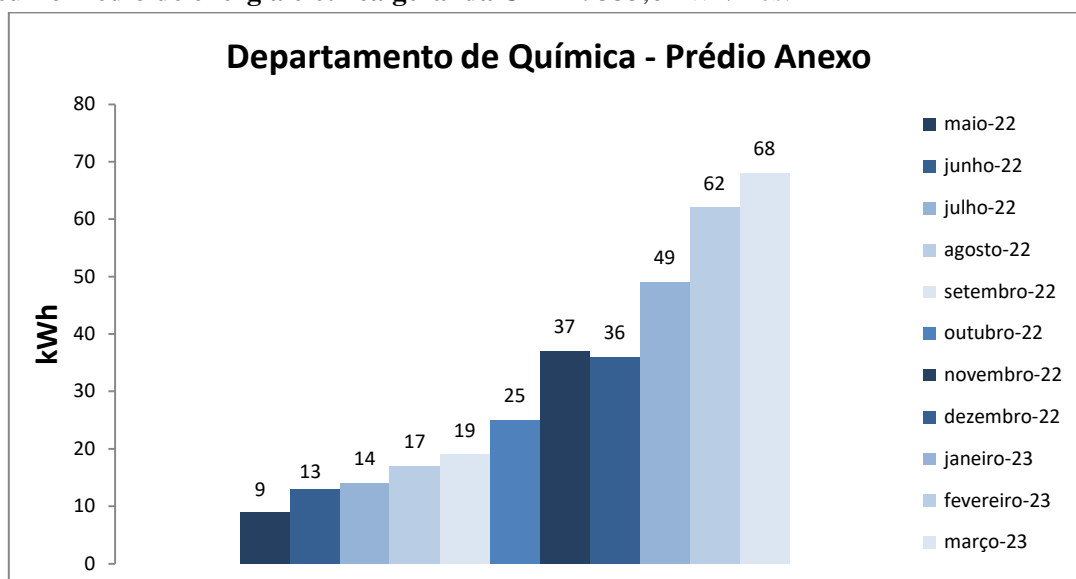
Figura 1. Variação do consumo de energia elétrica da edificação do Departamento de Química - prédio anexo
