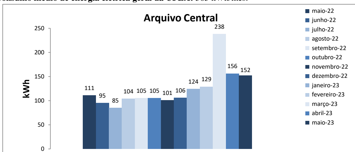
Figura 1. Variação do consumo de energia elétrica da edificação do Arquivo Central.
