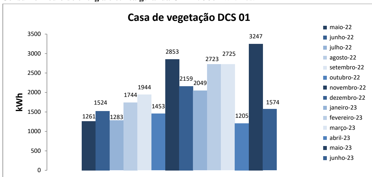
Figura 1. Variação do consumo de energia elétrica da edificação do Departamento de Ciência do Solo Casa de Vegetação 01
