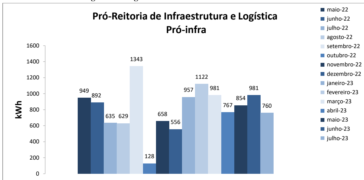
Figura 1. Variação do consumo de energia elétrica do prédio da Pró-Infra.
