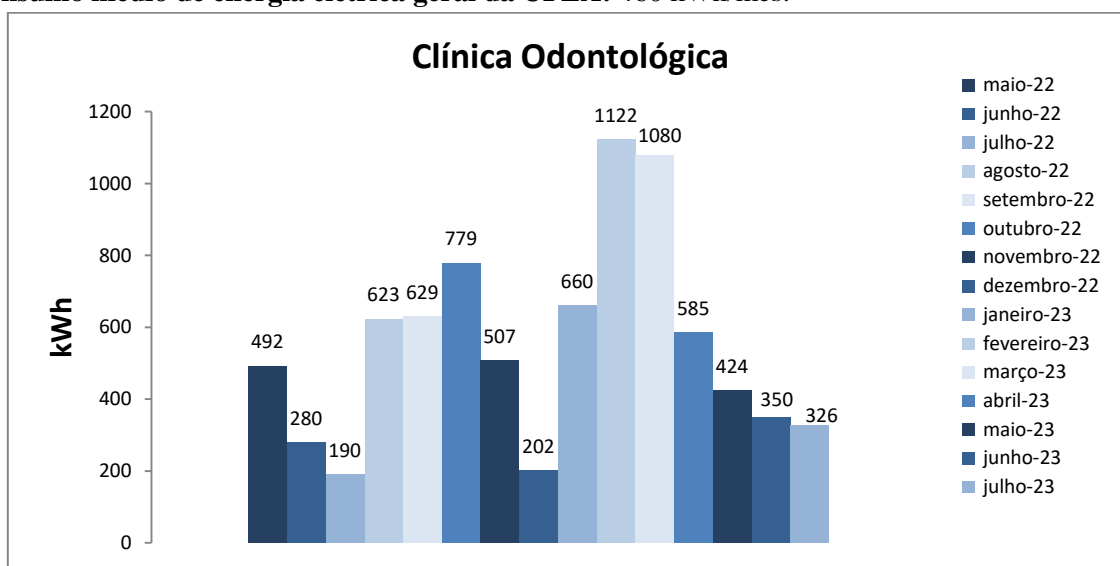
Figura 1. Variação do consumo de energia elétrica da edificação da Clínica Odontológica - PRAEC
