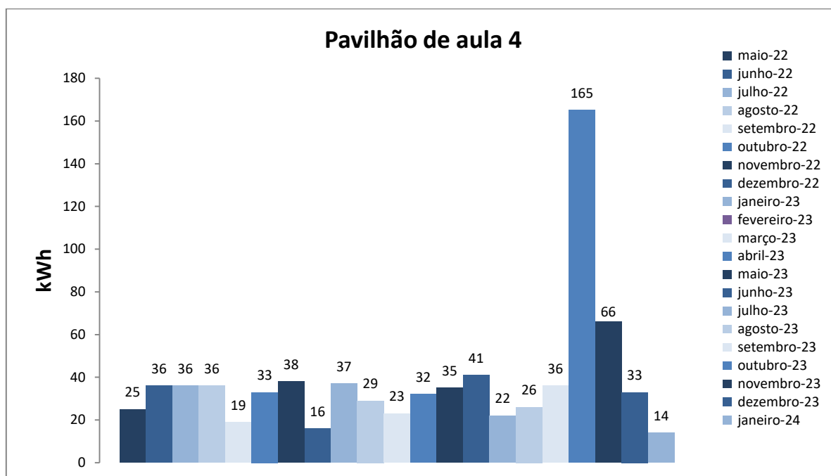
Figura 1. Variação do consumo de energia elétrica da edificação do Pavilhão de Aulas 04.
