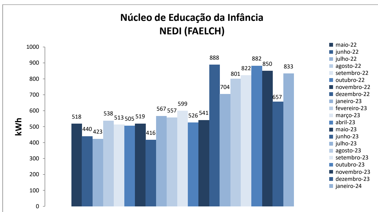
Figura 1. Variação do consumo de energia elétrica da edificação do Núcleo de Educação da Infância - NEDI.
