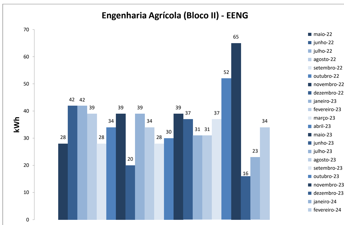
Figura 1. Variação do consumo de energia elétrica da edificação Engenharia Agrícola bloco II.
