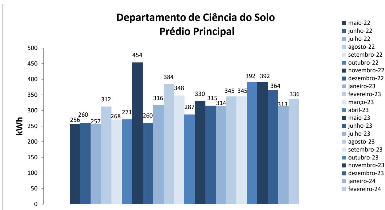
Figura 1. Variação do consumo de energia elétrica da edificação do Departamento de Ciência do Solo
