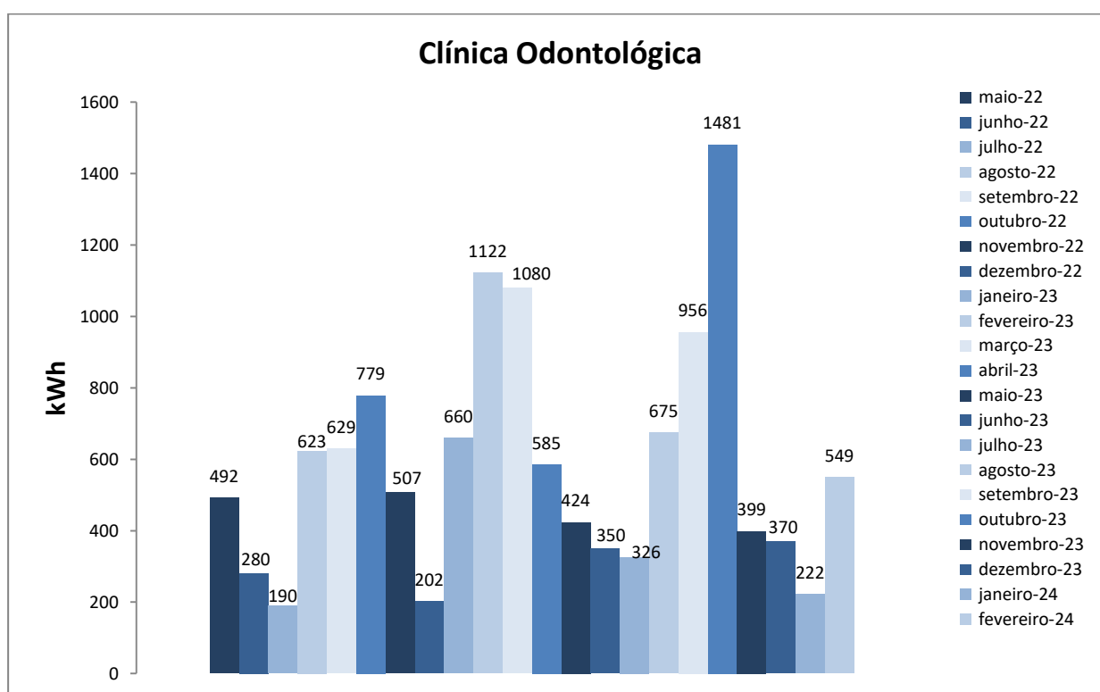
Figura 1. Variação do consumo de energia elétrica da edificação da Clínica Odontológica – PRAEC
