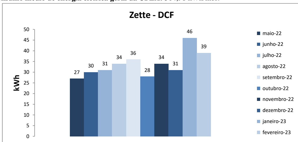
Figura 1. Variação do consumo de energia elétrica do prédio Zetta.
