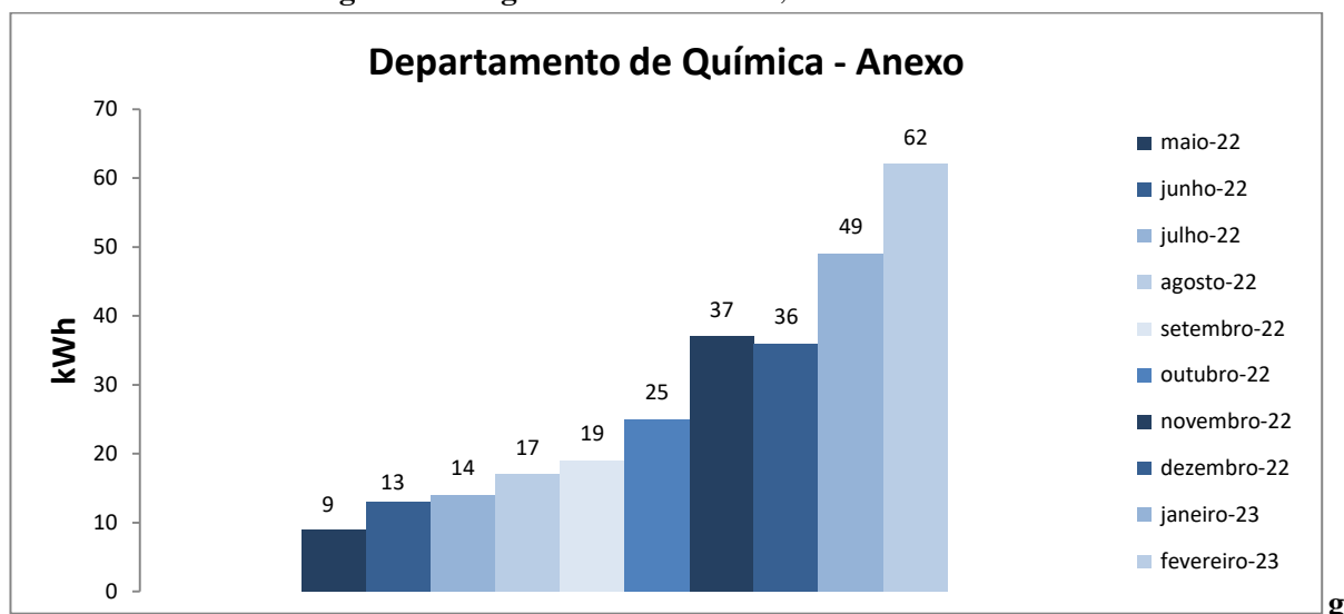
Figura 1. Variação do consumo de energia elétrica da edificação do Departamento de Química - prédio anexo
