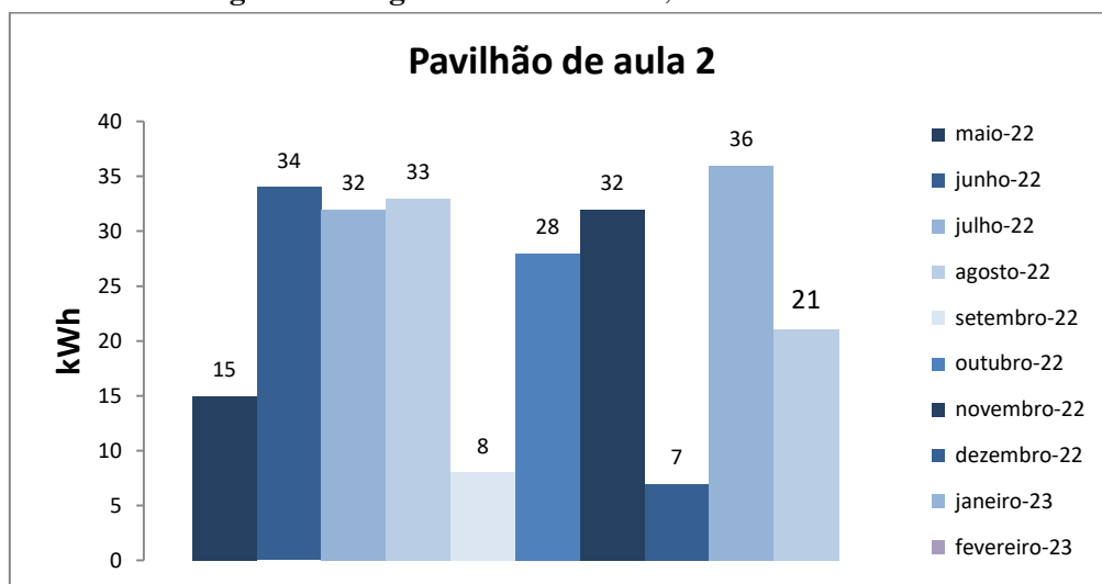
Figura 1. Variação do consumo de energia elétrica da edificação do Pavilhão de Aulas 02.
