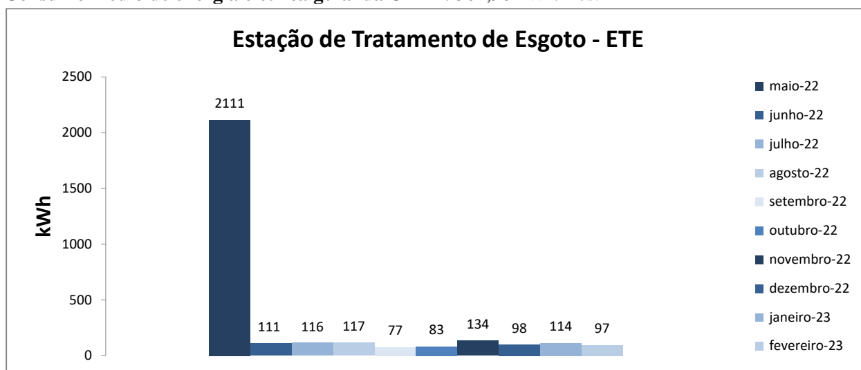
Figura 1. Variação do consumo de energia elétrica da Estação de Tratamento de Esgoto – ETE.
