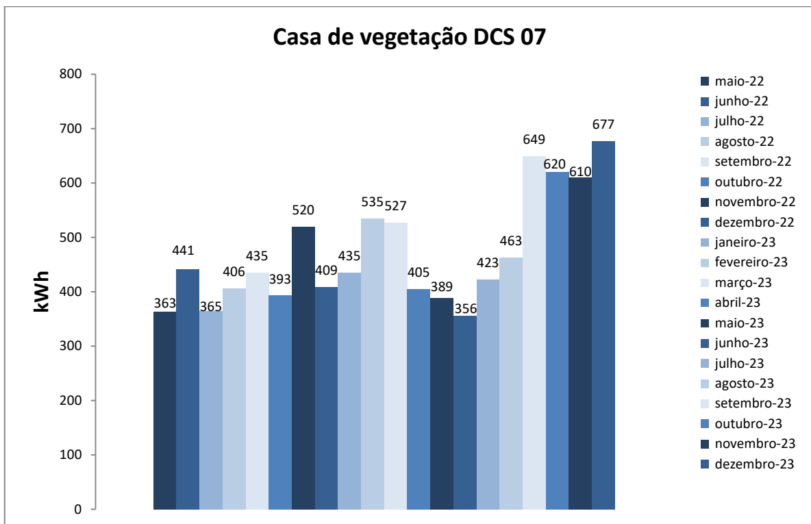
Figura 1. Variação do consumo de energia elétrica da edificação do Departamento de Ciência do Solo Casa de Vegetação 07
