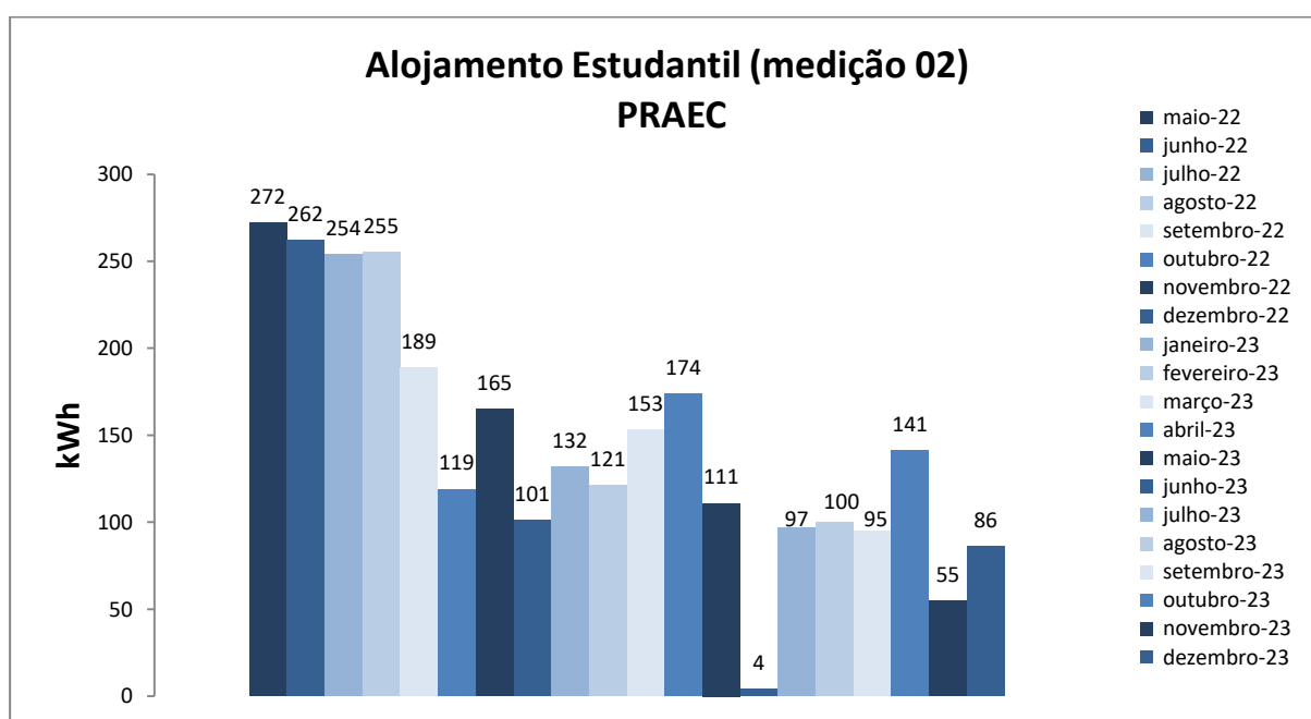
Figura 1. Variação do consumo de energia elétrica da edificação do Alojamento Estudantil – medição 02.
