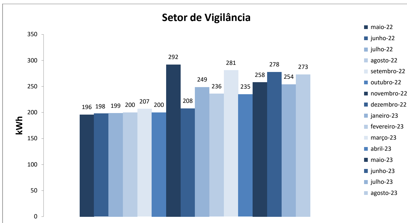
Figura 1. Variação do consumo de energia elétrica da edificação do Setor de Vigilância.
