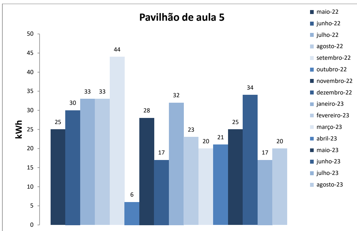
Figura 1. Variação do consumo de energia elétrica da edificação do Pavilhão de Aulas 05.
