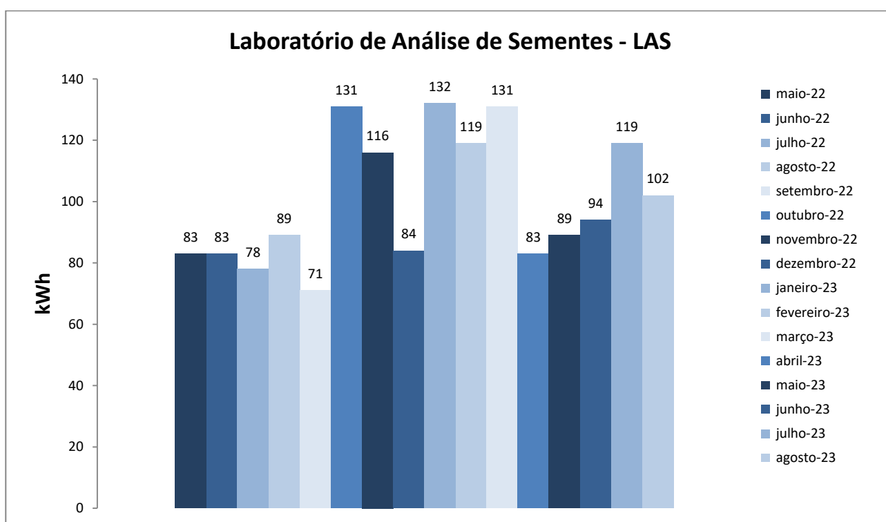
Figura 1. Variação do consumo de energia elétrica das edificações do Laboratório de Análise de Sementes.
