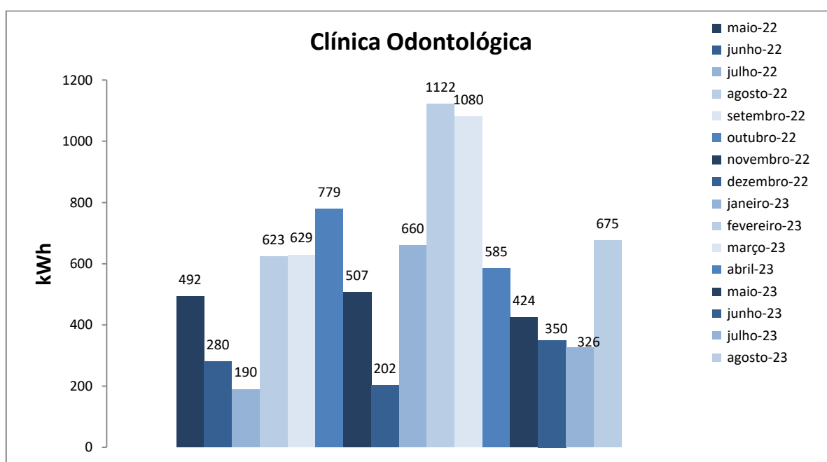
Figura 1. Variação do consumo de energia elétrica da edificação da Clínica Odontológica – PRAEC
