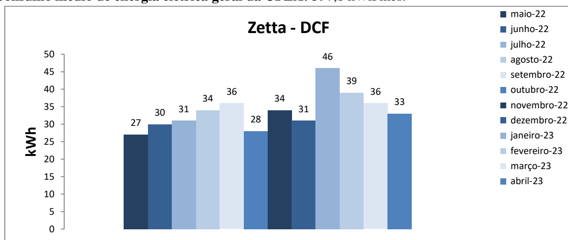
Figura 1. Variação do consumo de energia elétrica do prédio Zetta.
