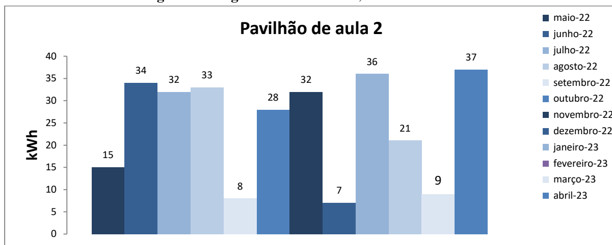
Figura 1. Variação do consumo de energia elétrica da edificação do Pavilhão de Aulas 02.
