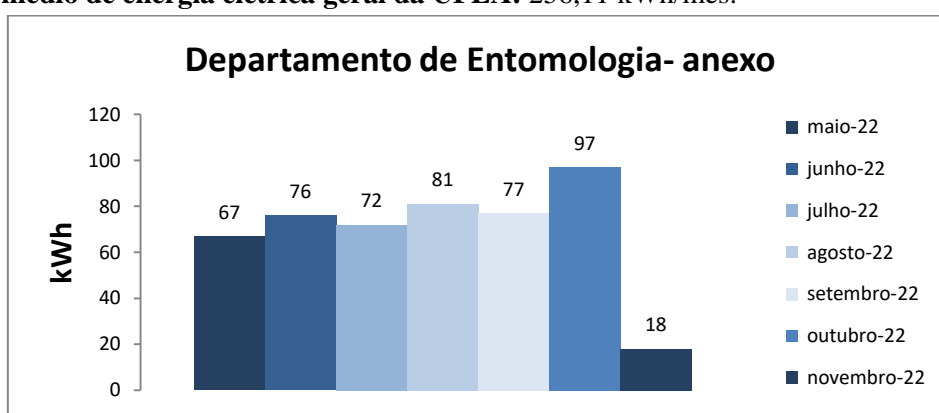
Figura 1. Variação do consumo de energia elétrica da edificação do Departamento de Entomologia Prédio anexo
