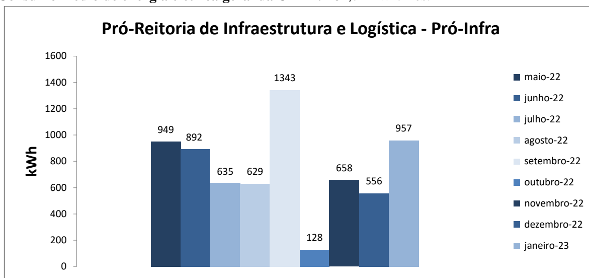
Figura 1. Variação do consumo de energia elétrica do prédio da Pró-Infra.
