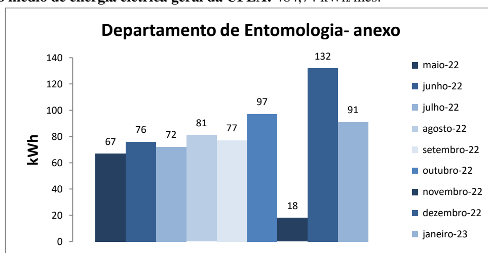
Figura 1. Variação do consumo de energia elétrica da edificação do Departamento de Entomologia Prédio anexo
