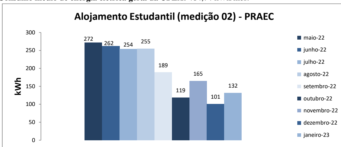
Figura 1. Variação do consumo de energia elétrica da edificação do Alojamento Estudantil – medição 02.
