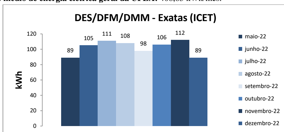
Figura 1. Variação do consumo de energia elétrica da edificação do Departamento de Exatas
