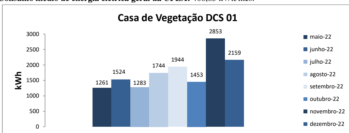
Figura 1. Variação do consumo de energia elétrica da edificação do Departamento de Ciência do Solo Casa de Vegetação 01
