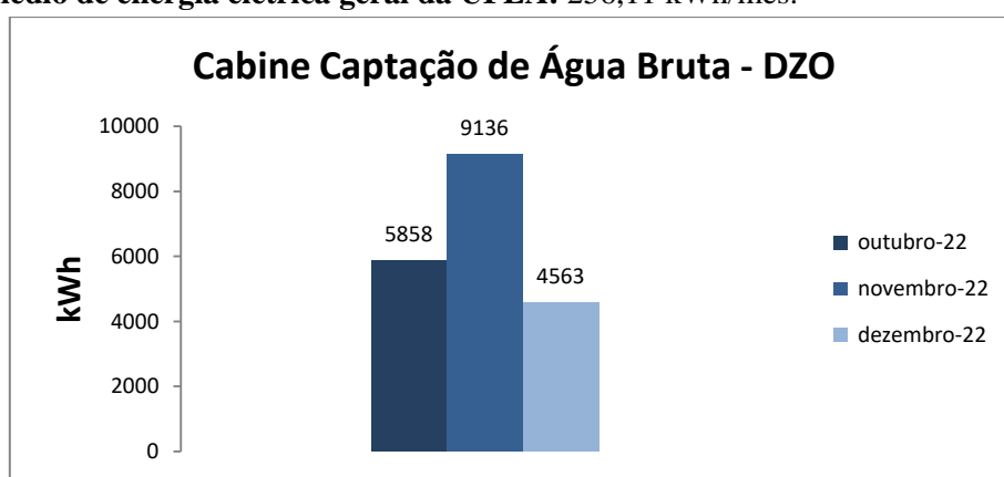
Figura 1. Variação do consumo de energia elétrica da Cabine Barragem Captação Água Bruta - DZO.
