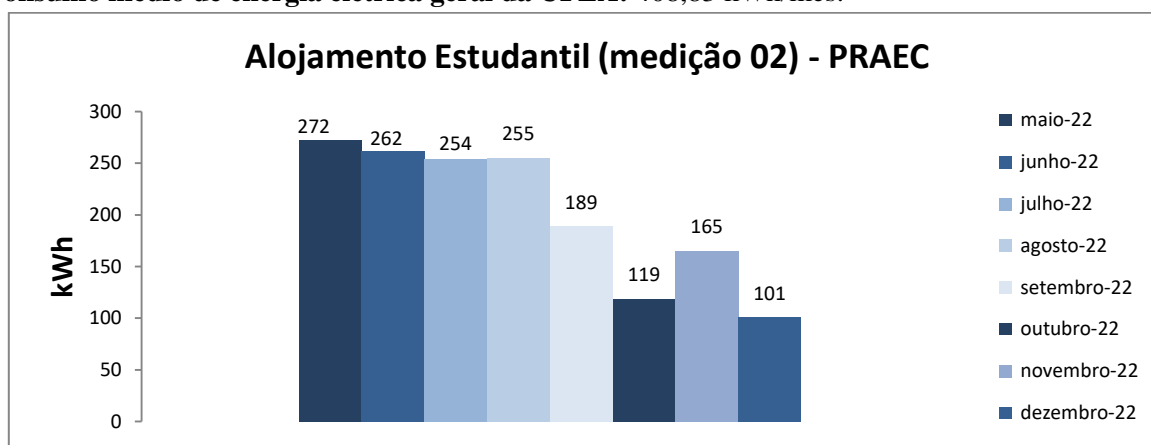
Figura 1. Variação do consumo de energia elétrica da edificação do Alojamento Estudantil – medição 02.
